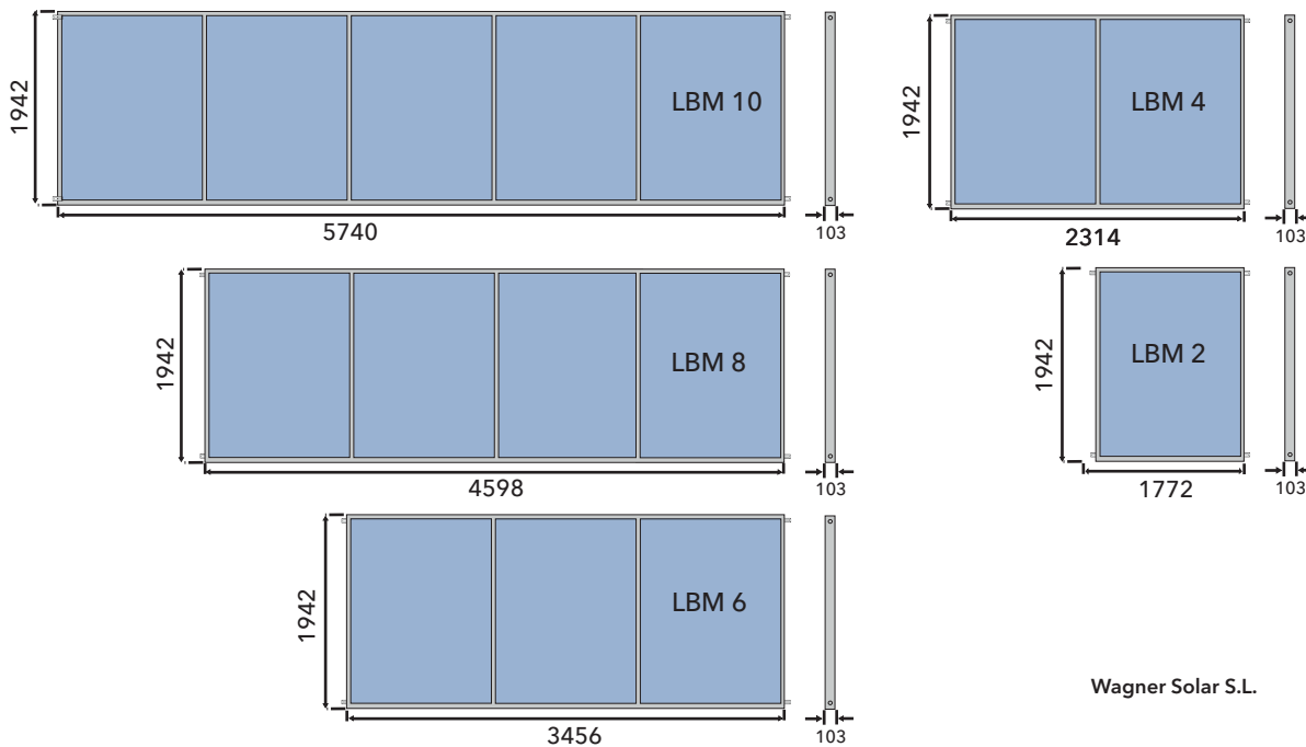
Fig 2 Dimensiones del captador LBM
